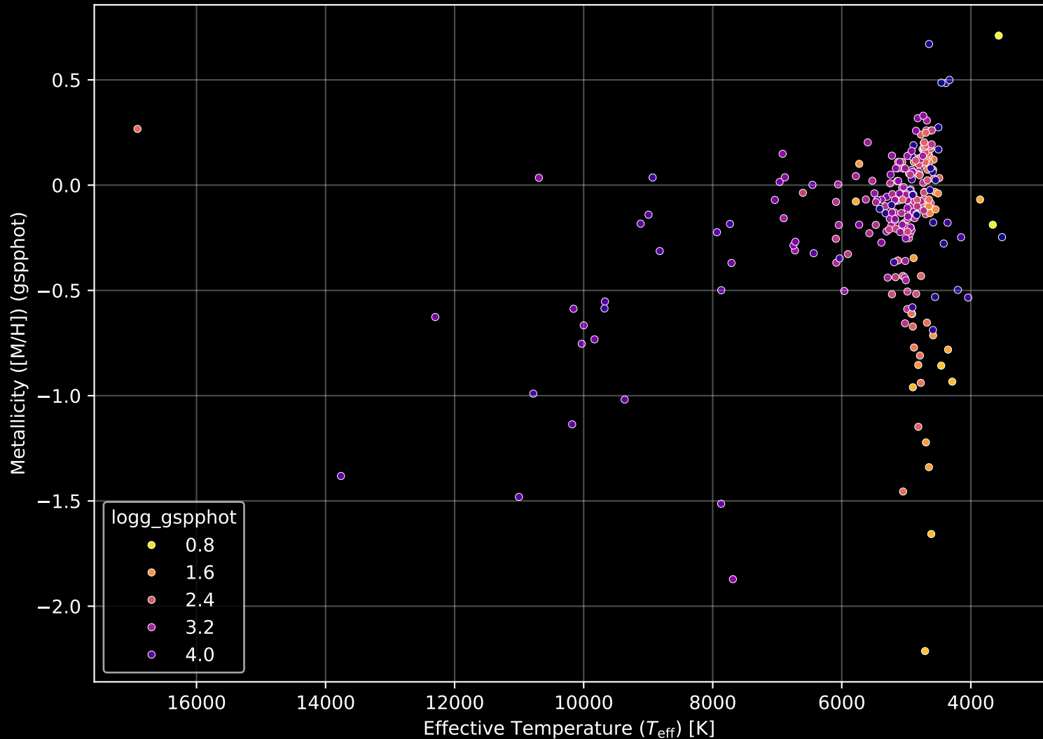
APOGEE DR17 Field: [109+12] Stellar Population Parameters (n= 268)
